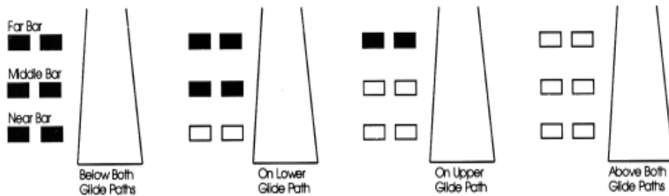
FIG 2-1-3 3-Bar VASI
