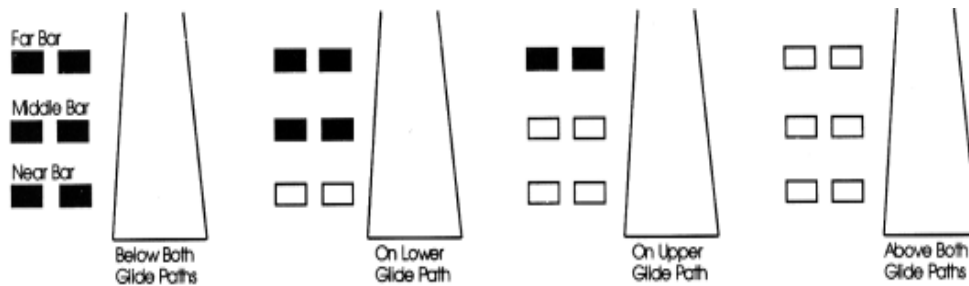
FIG 2-1-3 3-Bar VASI
